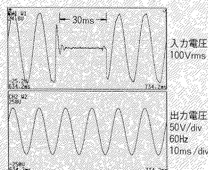
瞬停時の出力電圧波形
